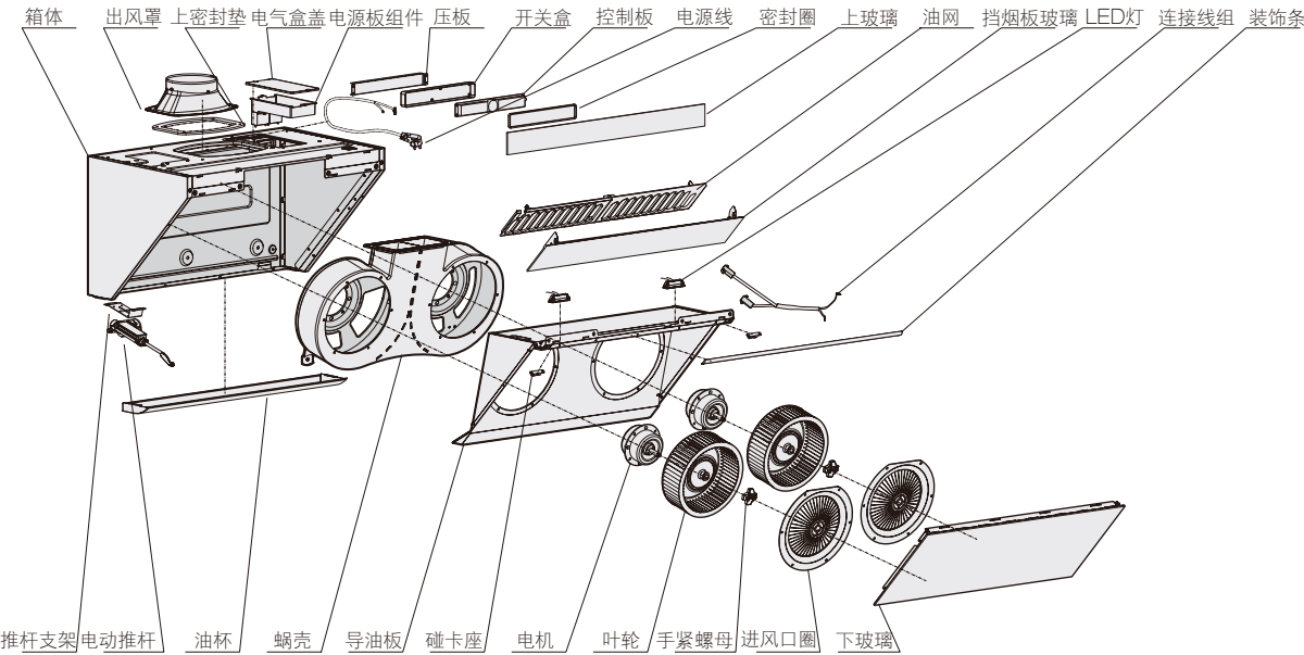
爆炸图
