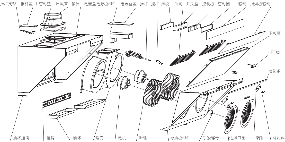
爆炸图
