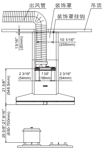
图 3 安装示意图
